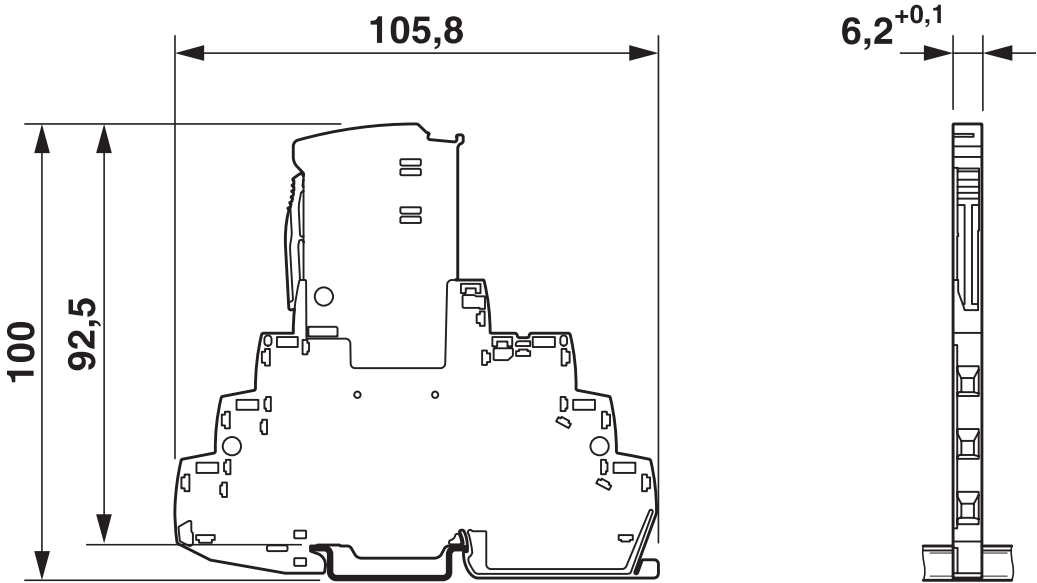
尺寸图
