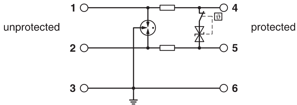
电路图
