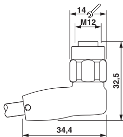
外形寸法
