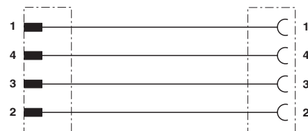
回路図
