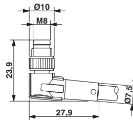
外形寸法
