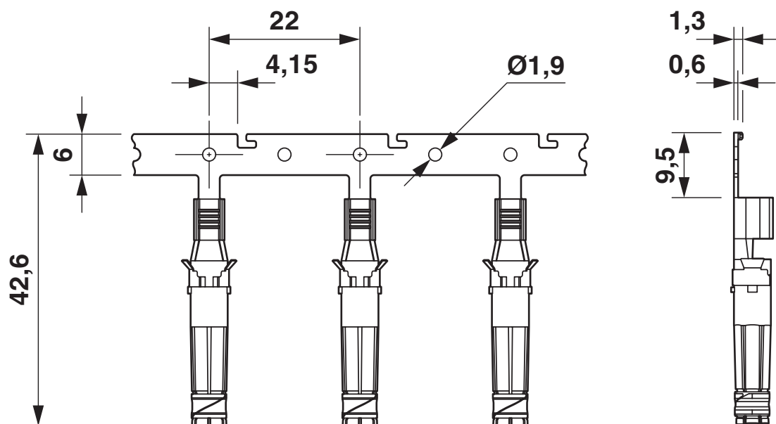
尺寸图
