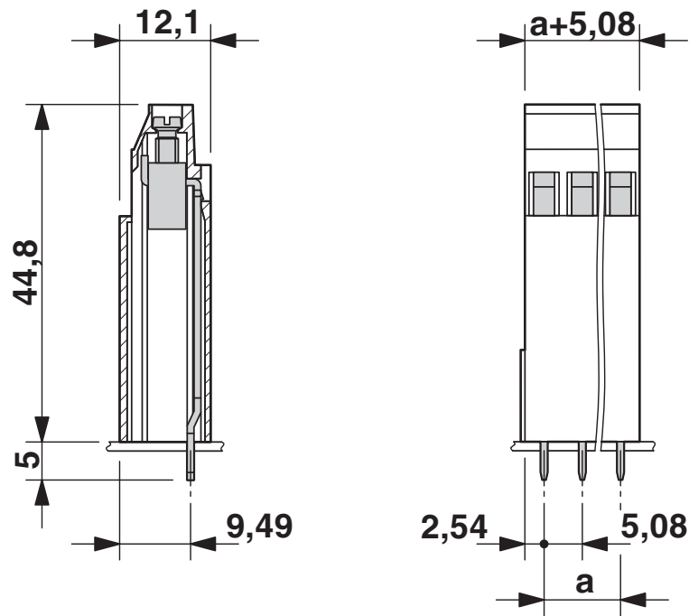
尺寸图
