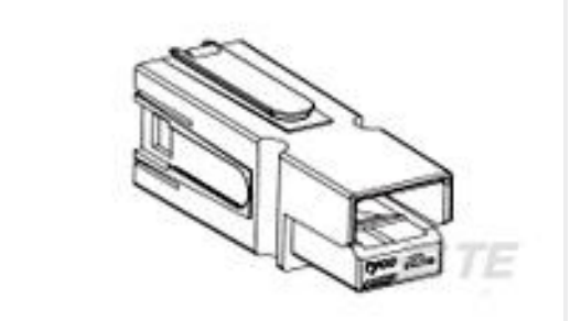
TE Part #1445715-9 75A HSG SUBASY GREEN
