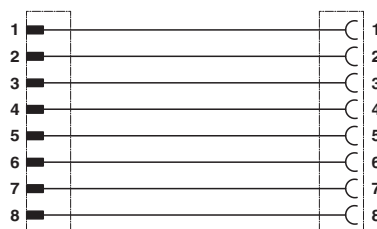
回路図
