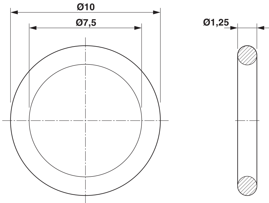
尺寸图
