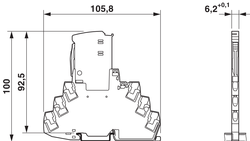
尺寸图
