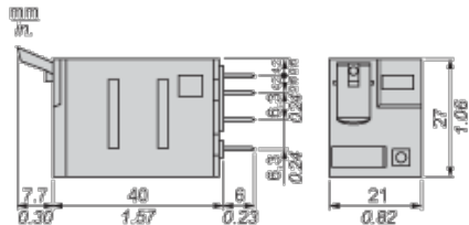
Stecker-Seitenansicht
