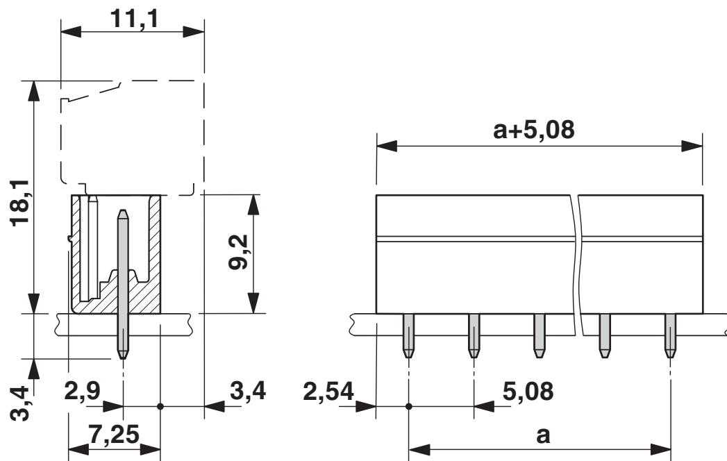
尺寸图
