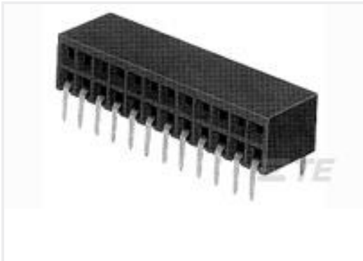
TE Part #4-87962-2 86 MODII HORZ DR CE 100CL/115
