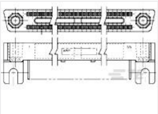
TE Part #443851-1 MINI BOX RCPT ASSY/MTG EARS
