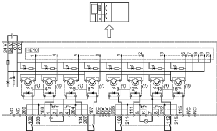
接线图
