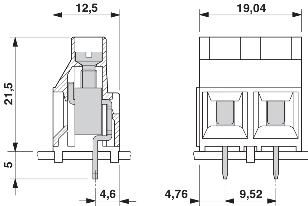
尺寸图
