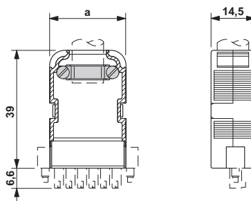
Dessin coté
