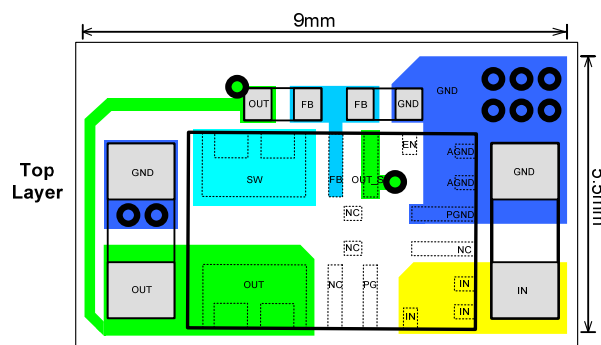
Figure 3— Top Layer
