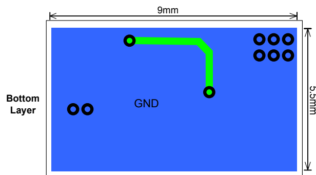
Figure 4— Bottom Layer
