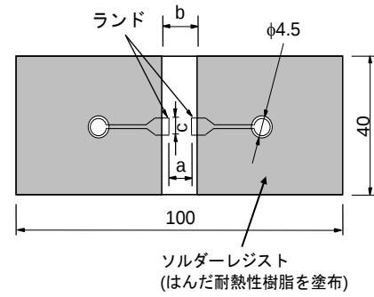
図1 (単位:mm)
