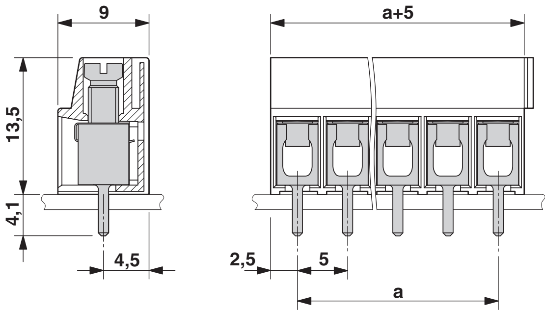
尺寸图
