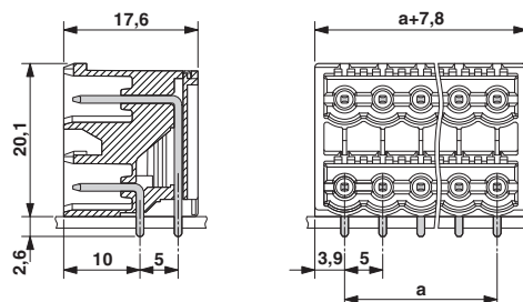
外形寸法
