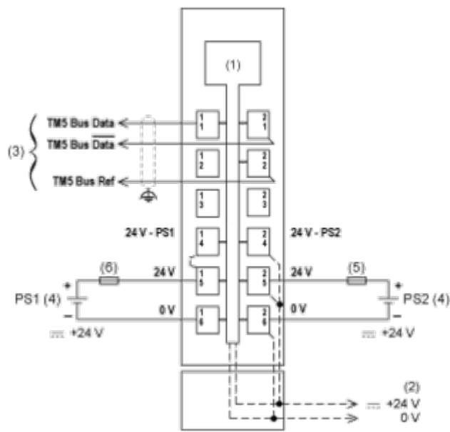
接线图
