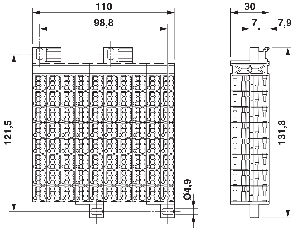
尺寸图
