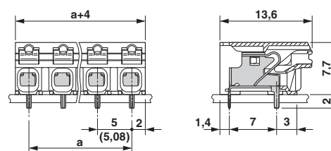
外形寸法
