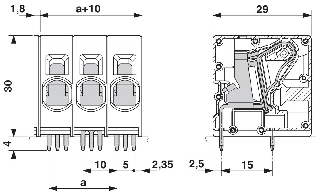
尺寸图
