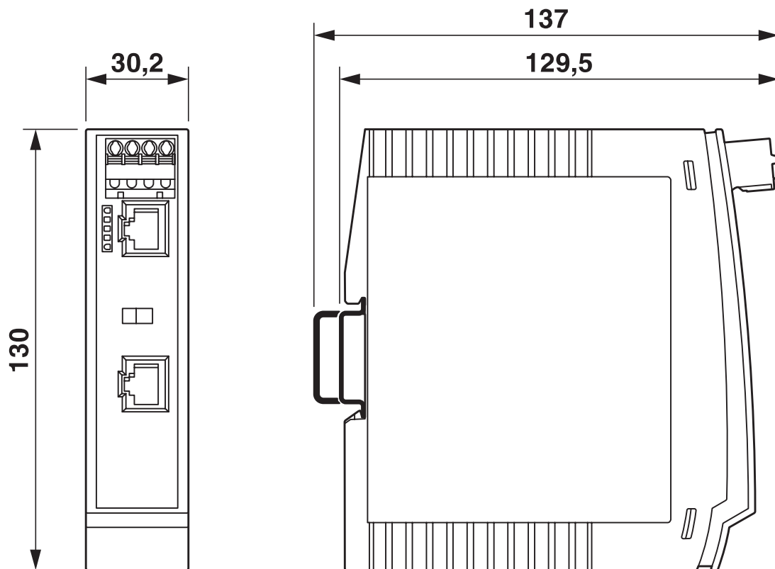
尺寸图
