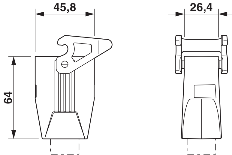
尺寸图
