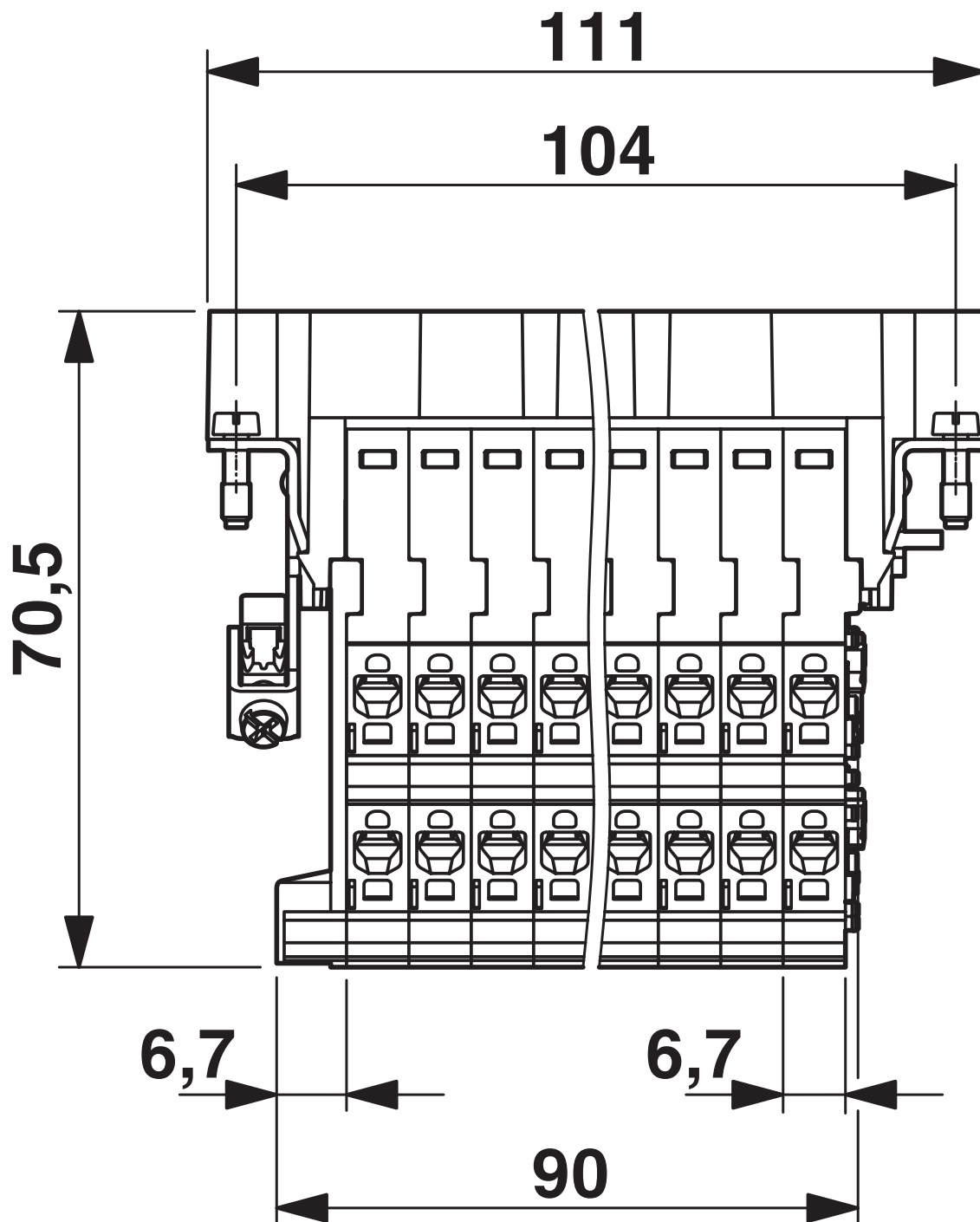
尺寸图
