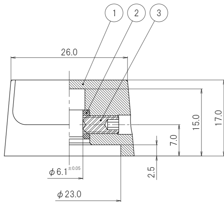
A-O-A' SECTION
