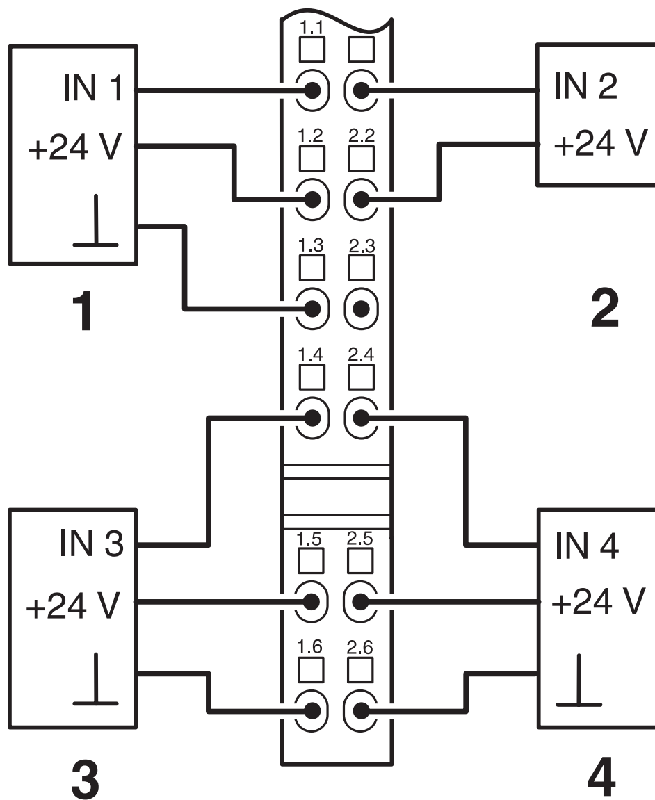
接线图
