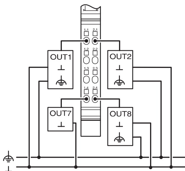
接线图
