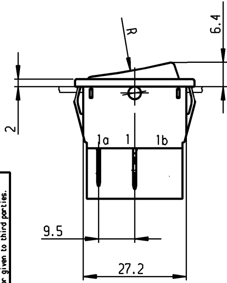
Flachstecker plug-in DIN 46244-A6.3x0.8
