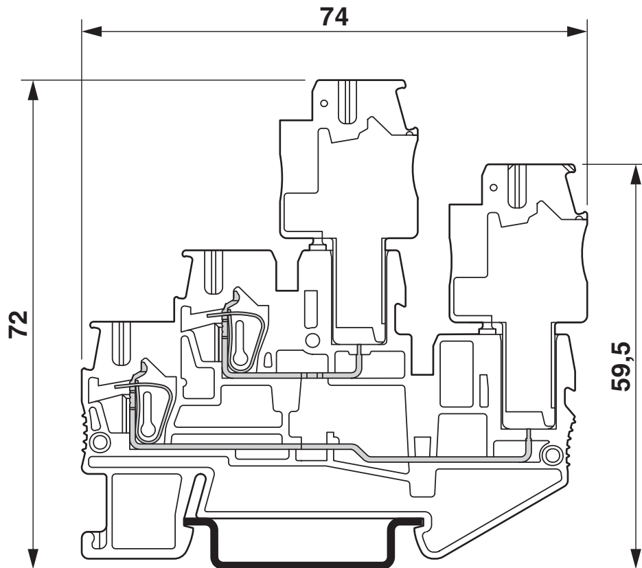
尺寸图
