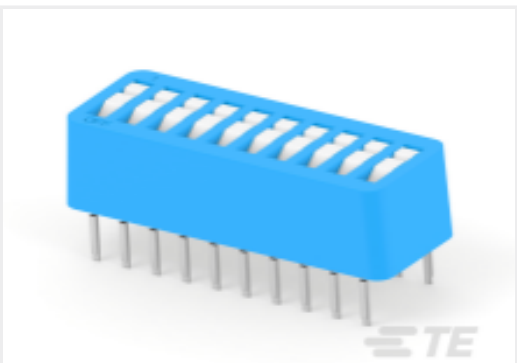
TE Part # 3-435668-0 DIP SW 10 POSN W/TAPE AU
