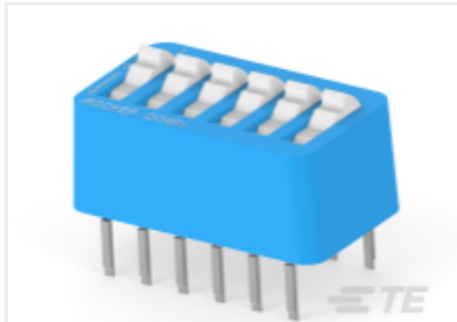
TE Part # 5435640-4 DIP SW 6POSN AU
