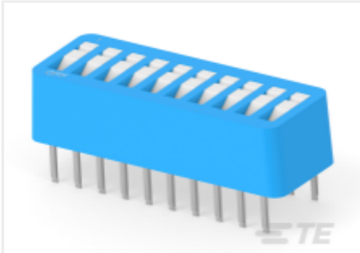
TE Part # 3-5435668-0 DIP SW 10 POSN W/TAPE AU
