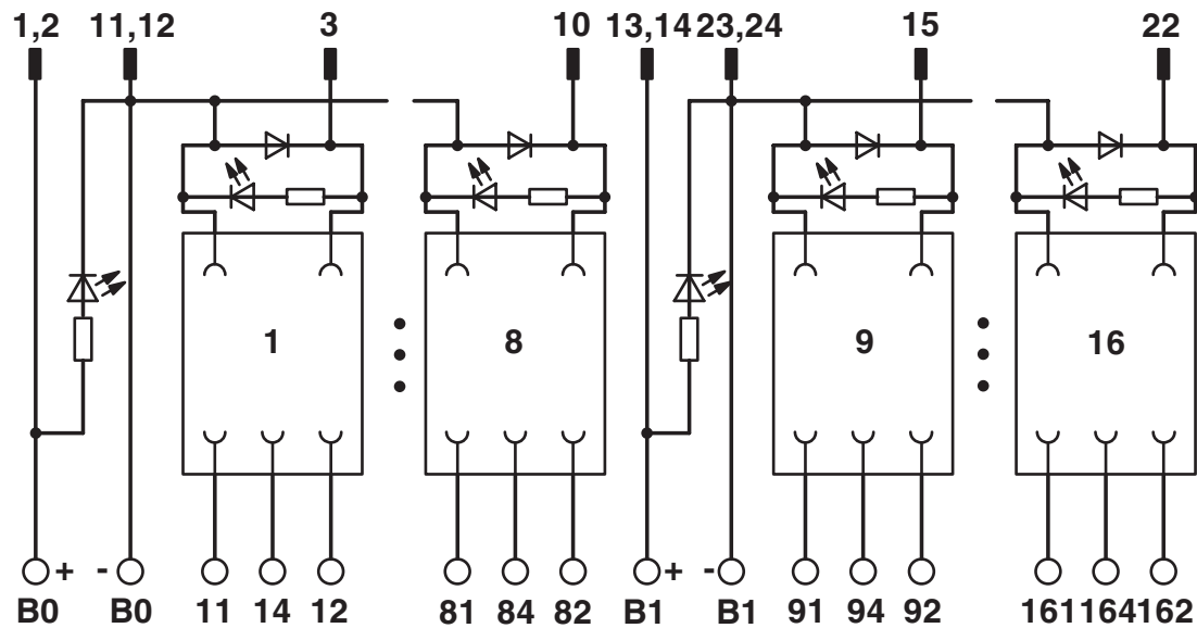
Schaltplan
