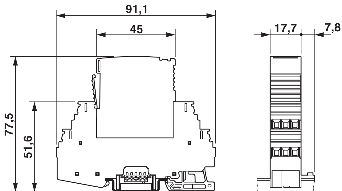
尺寸图
