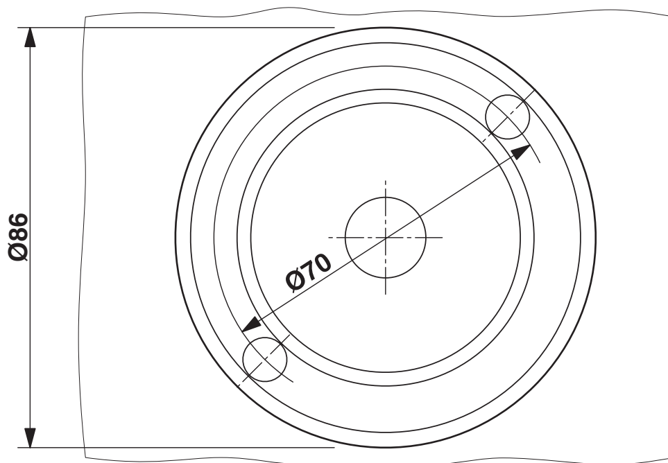
Bohrplan/Lötpadgeometrie
