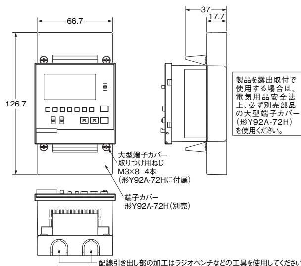
〈大型端子カバー (別売) 取り付け時〉
