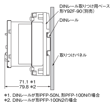
〈DINレール取り付け時〉
