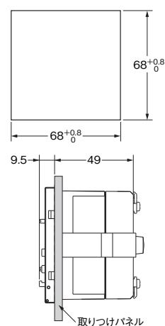
パネルカット寸法 (DIN43700準拠)
