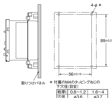
取り付け穴加工寸法
