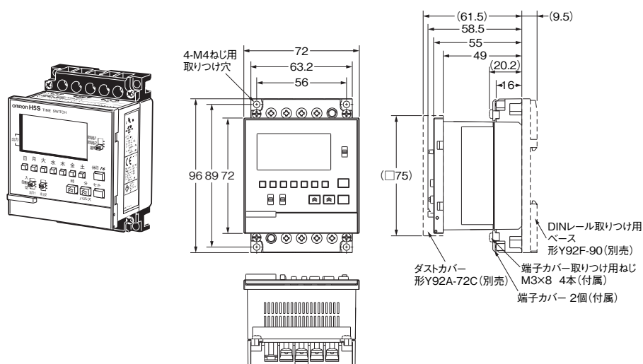
〈大型端子カバー (別売) 取り付け時〉
