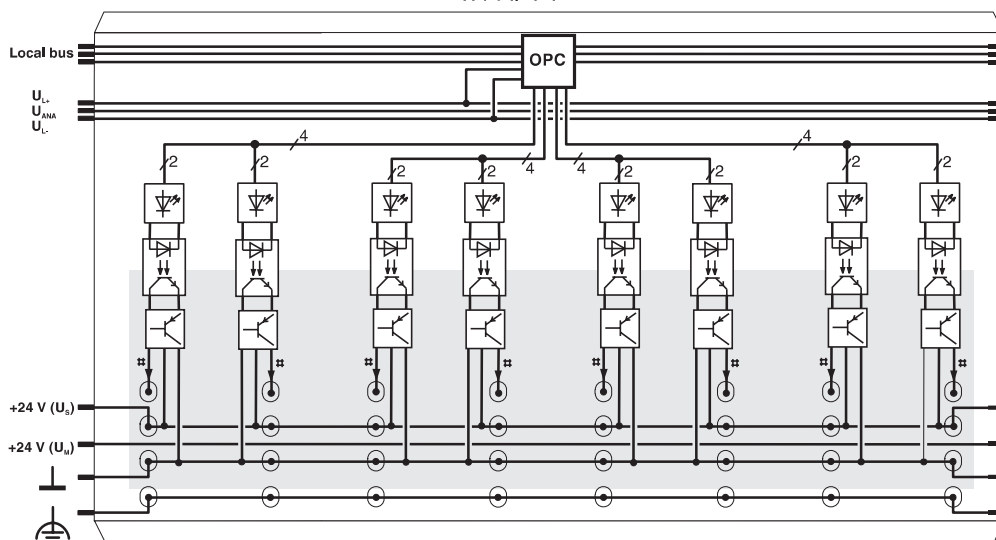
结构框图
