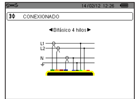
Figura 13: conexión bifásica de 4 hilos
