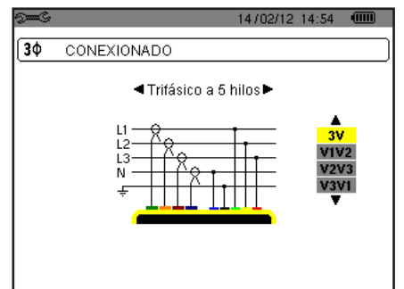
Figura 16: conexión trifásica de 5 hilos
