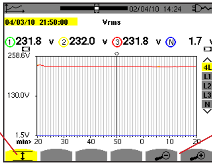
Figura 92: Vrms (4L) con MIN-AVG-MAX
