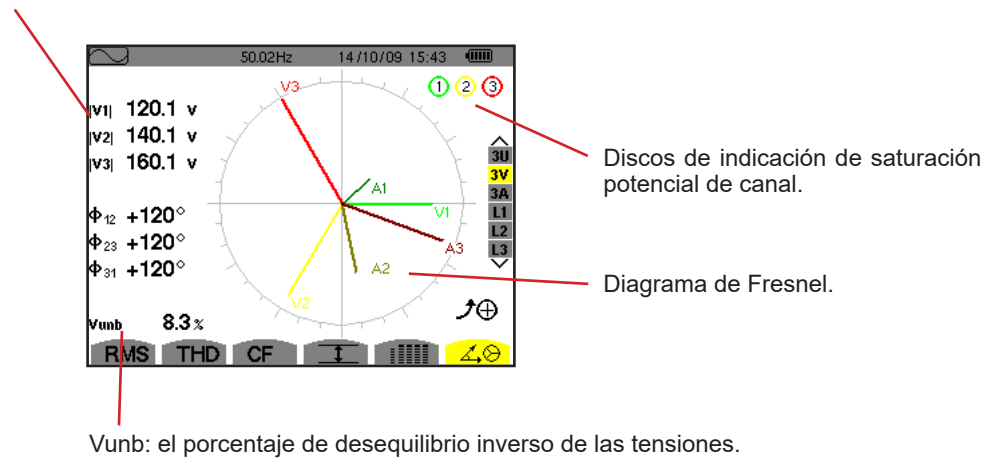
Figura 82: la pantalla de visualización del diagrama de Fresnel en 3V
