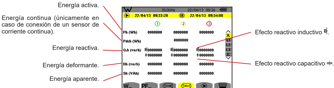
Figura 112: la pantalla de visualización de las energías aportadas en 3L
