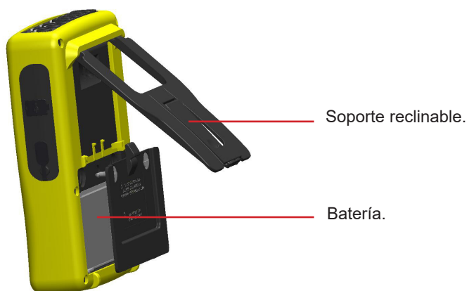
Figura 5: soporte y tapa de acceso a la batería
