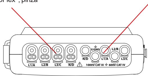
Figura 3: los bornes de conexión
