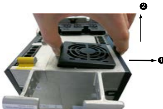
Figure 91: Removing the fan module
