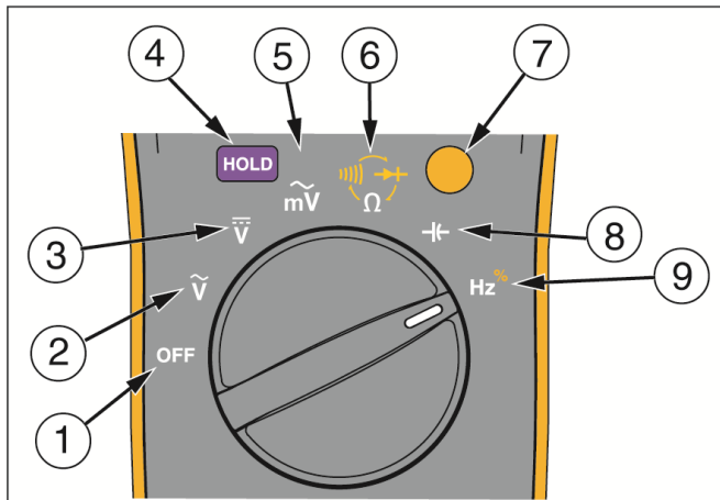
图 2. 旋转开关
