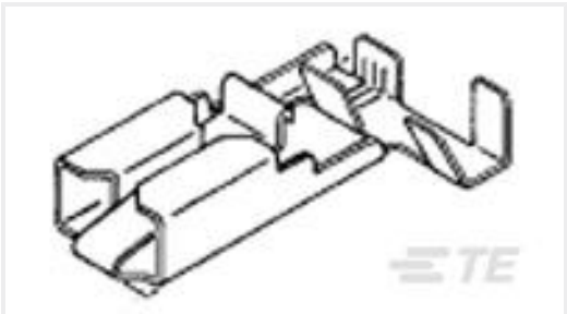
TE Part #926790-4 PL 250 FLAG REC 1-2.5 MM2 PTP CUZN30 F53
