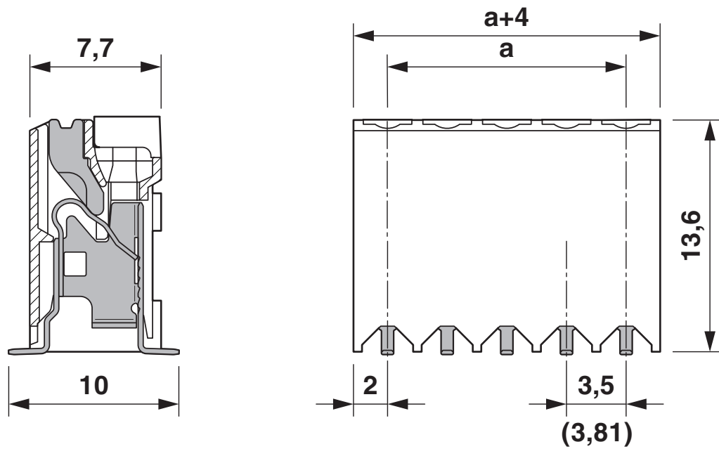
尺寸图
