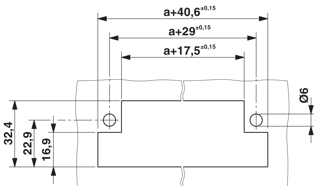
尺寸图
