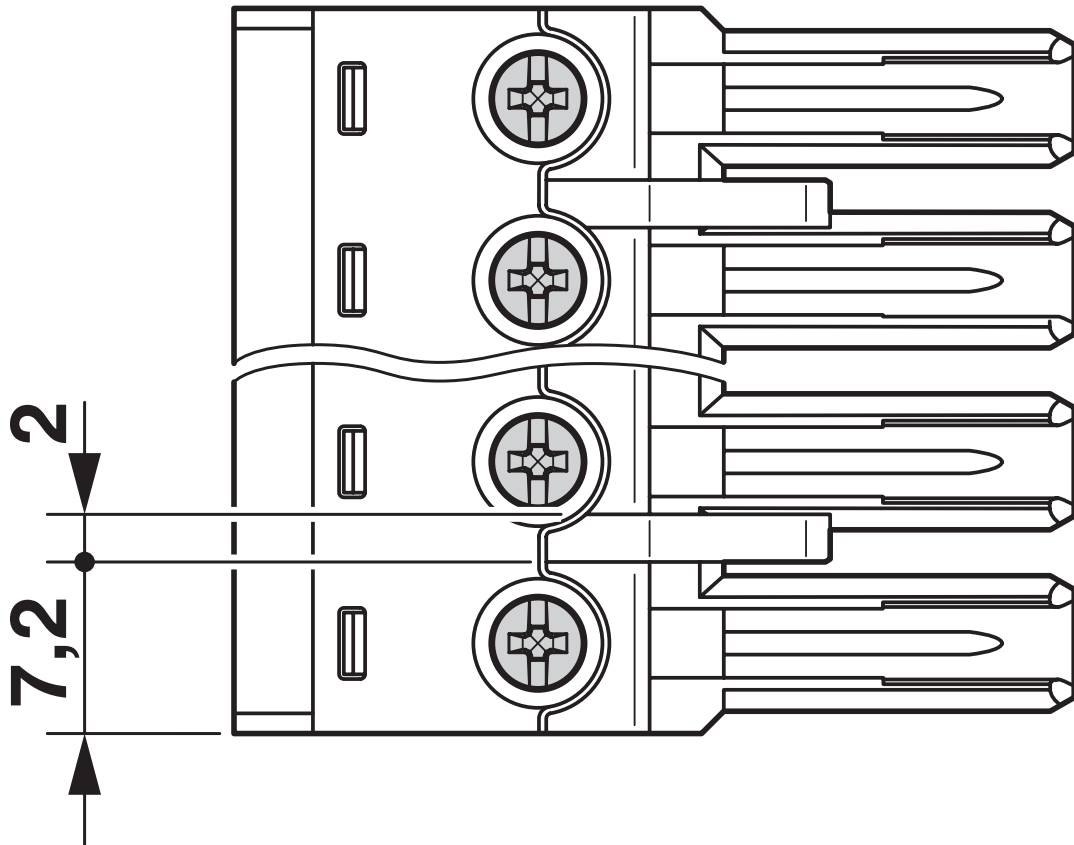
尺寸图
