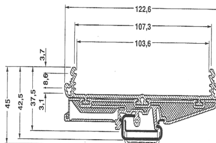
UM-108 PROFIL
