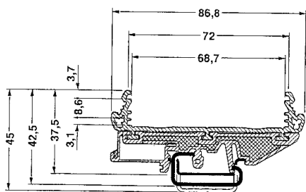
UM-72-PROFIL
