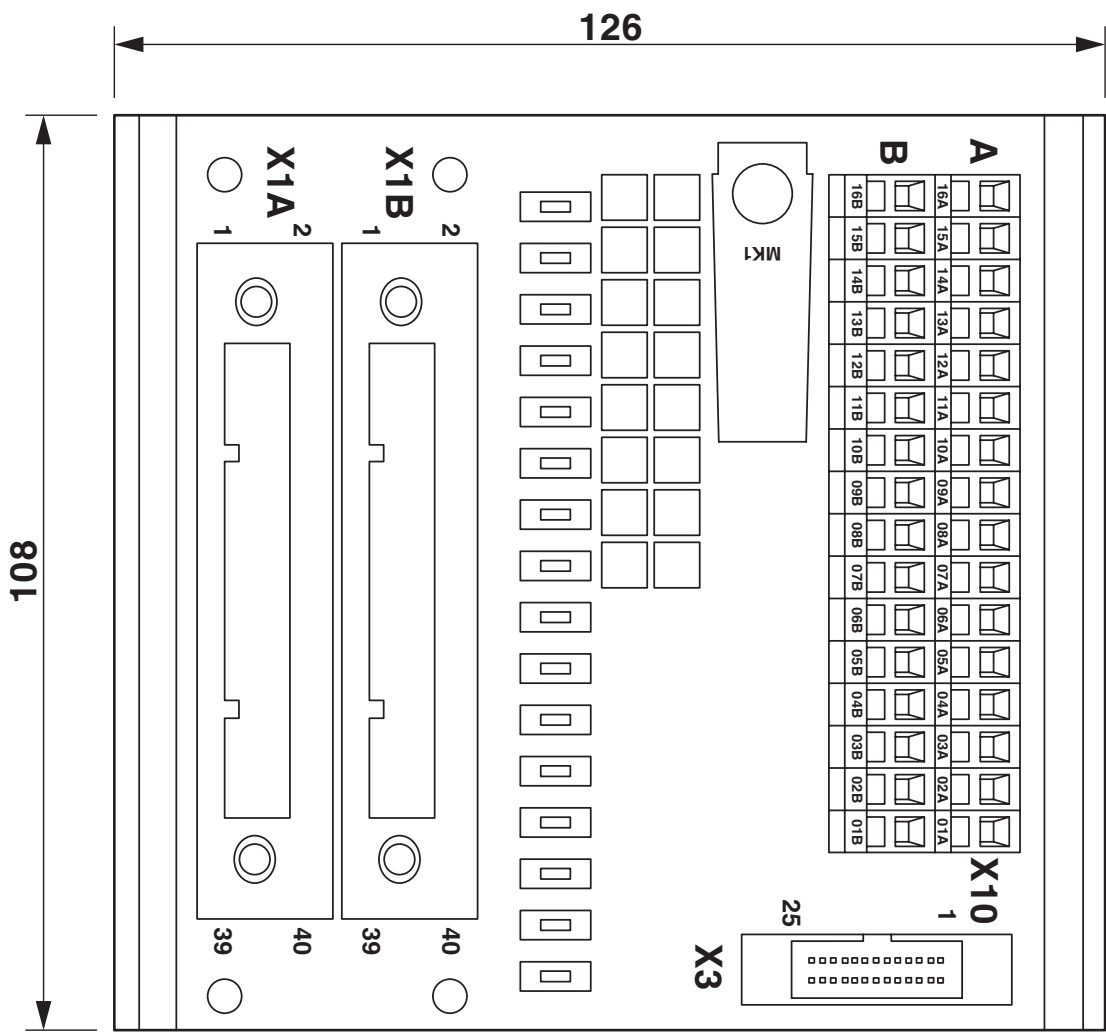
尺寸图
