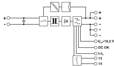
ブロック図
