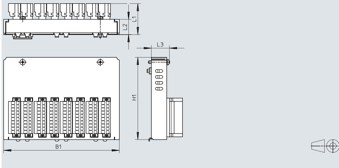
Dimensions – I/O module CDPX-EA-V1
