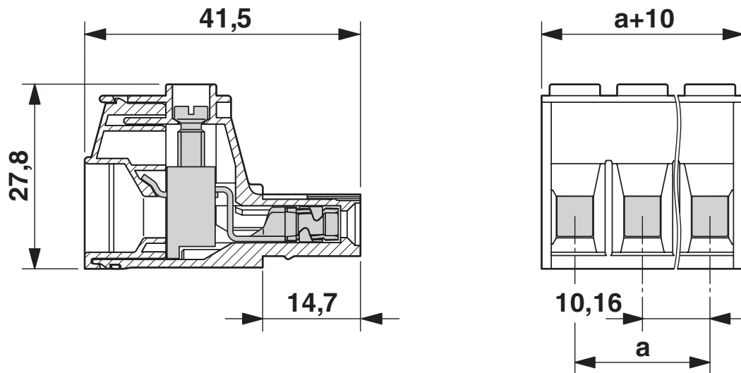
尺寸图
