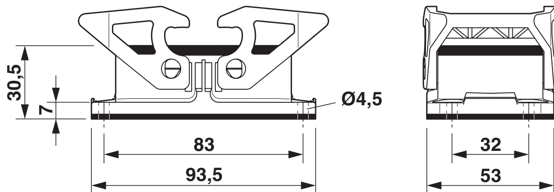
Maßzeichnung
